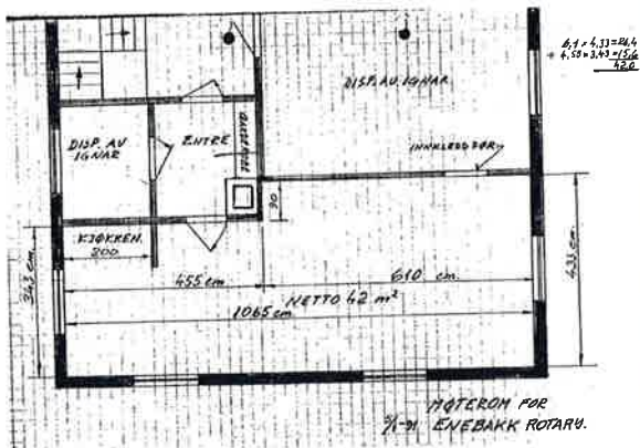
Planskisse over arbeidet.
